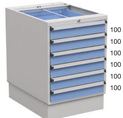
Bloc, hauteur 800 mm
