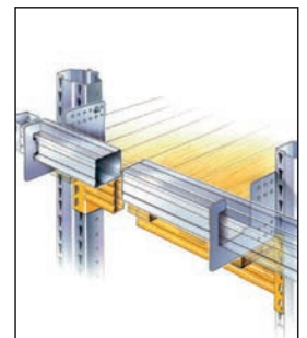
Butée de profondeur
